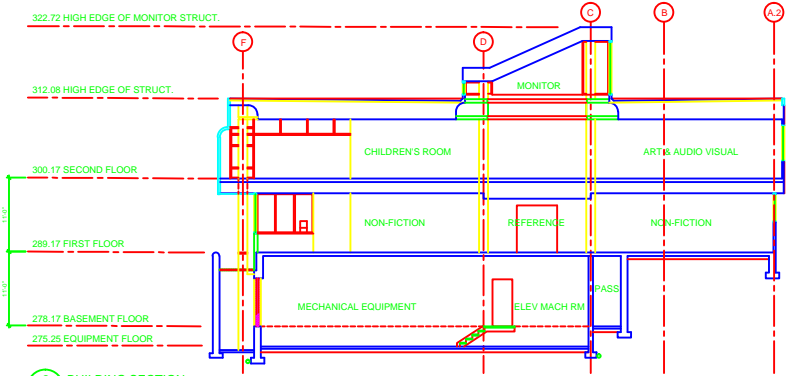
2 BUILDING SECTION A4 SCALE: 1/8" = 1'-0"
